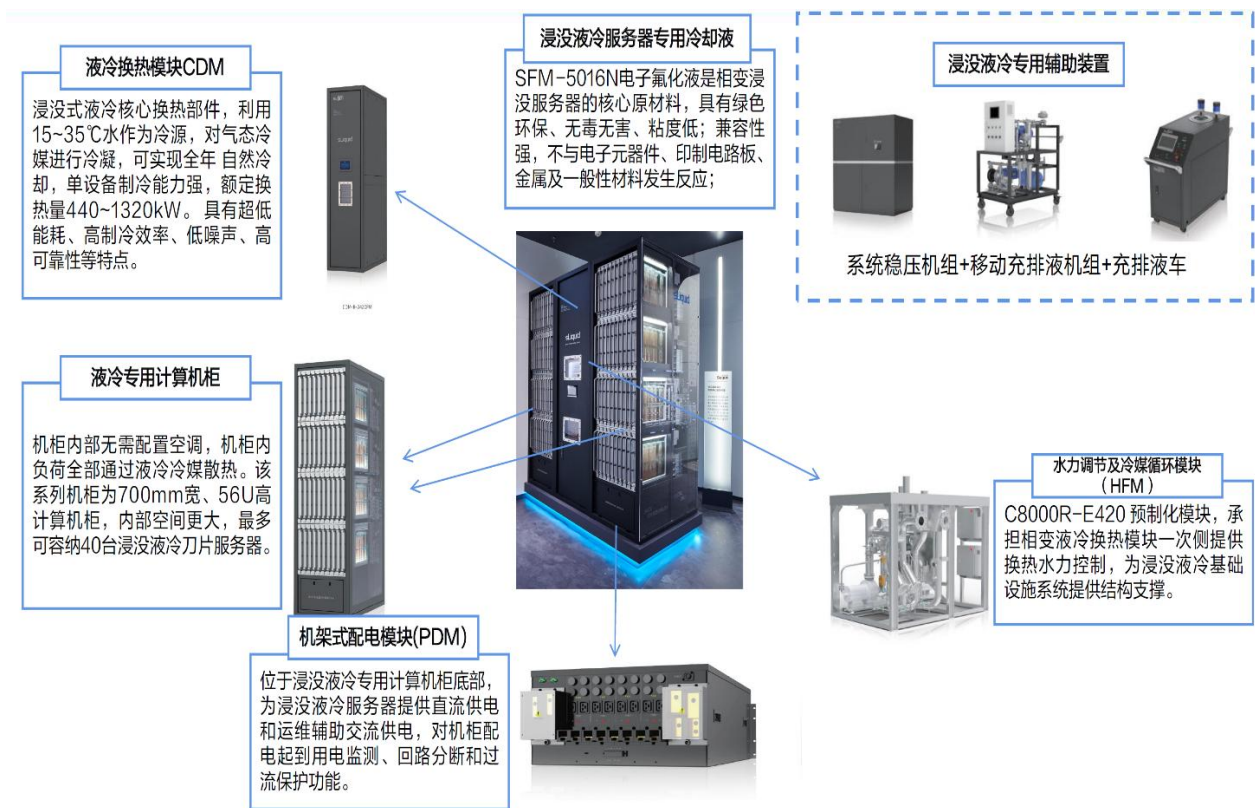
C8000 液冷机柜构成图
